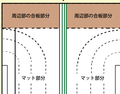
接着剤を塗布する位置
