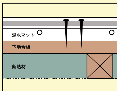
ステープルの打ち込み位置
