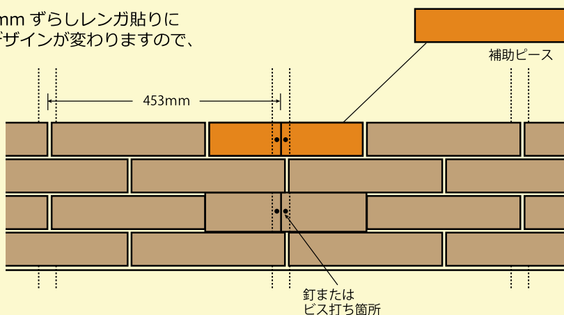
図2 補助ピースはめ込み
