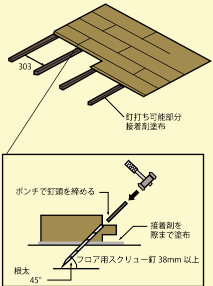
図 1：接着剤の塗布
