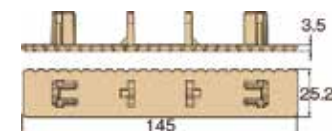
エンドキャップ
