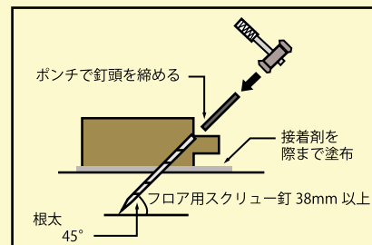
図 1：接着剤の塗布
