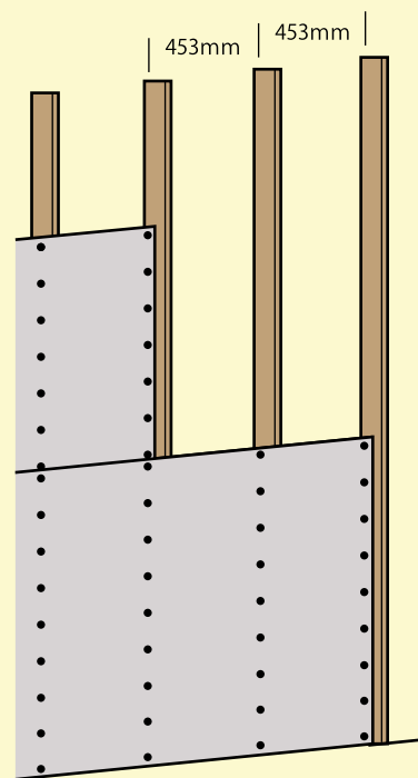
図1 下地の施工
