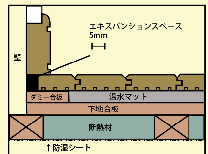
エキスパンションスペース
